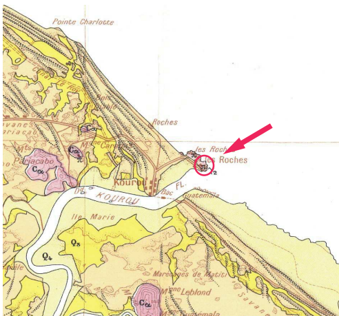
Carte géologique de Kourou à 1/100 000
